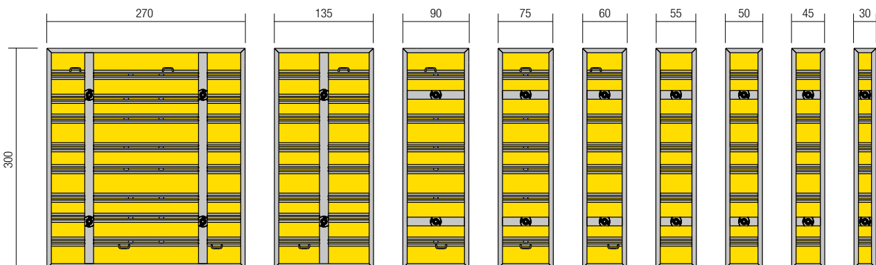
Elementraster von Framax Xlife plus 3,00 m / Angaben in cm
