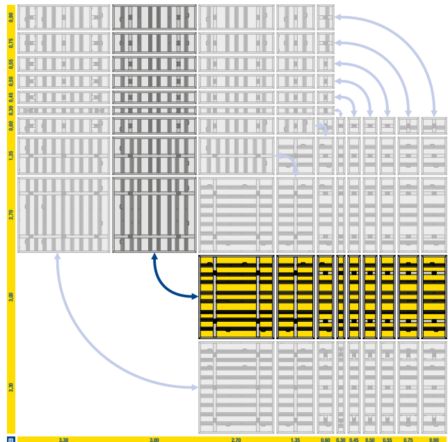
Elementhöhe 3,00 m: liegend und stehend mit allen Systemhöhen kombinierbar
