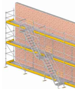
Fasadne skele
