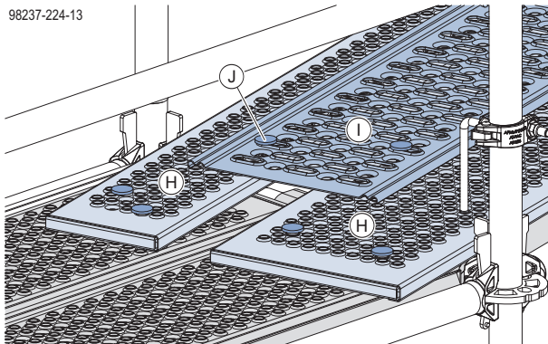
H Gap filler plank 19 or 32cm
