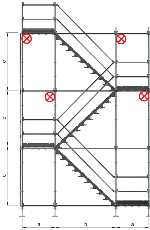
Elevation
