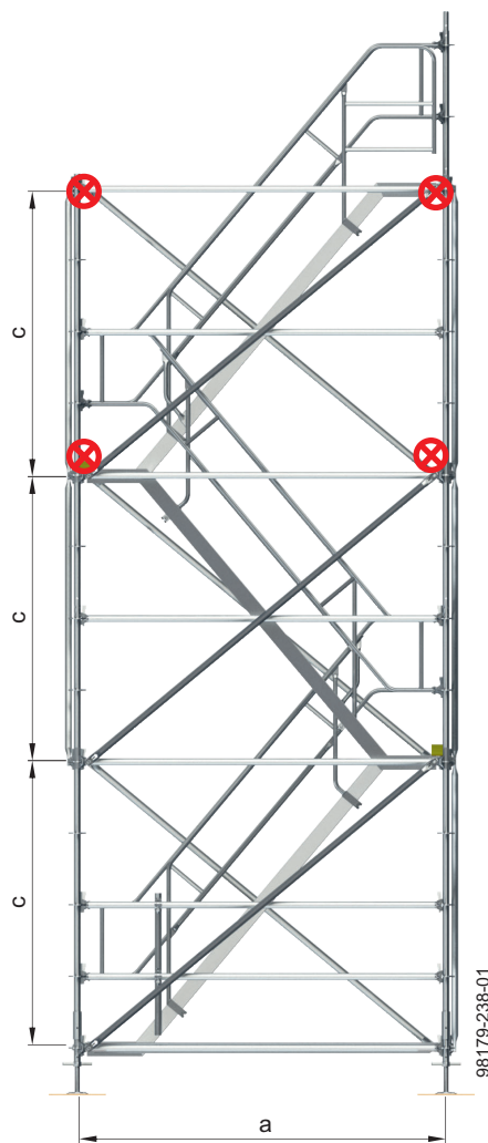
Elevation
