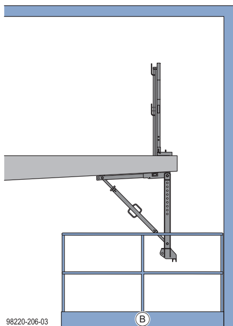
B Montagewagen
