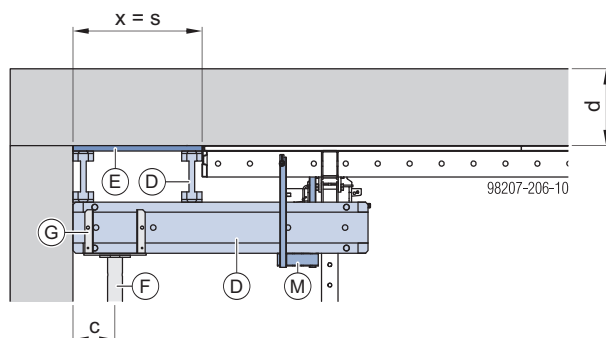
Einhängebügel im Funktionsprofil (zwischen Jochprofil und Rahmenprofil)
