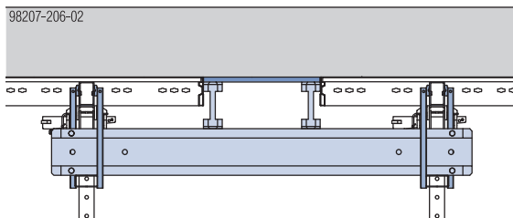
Einhängbügel ohne Zusatzunterstellung
