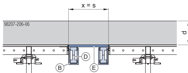
mit Trägeraufleger
