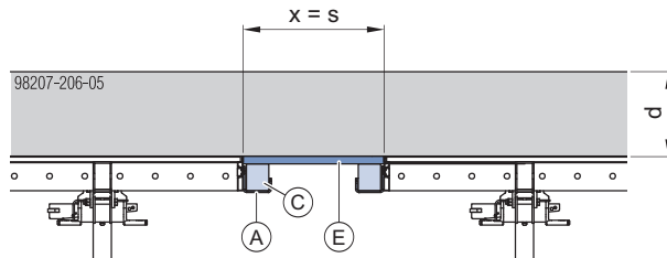
mit Kantholzaufleger
