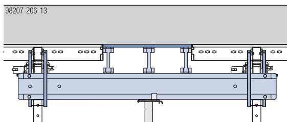
Einhängbügel mit Zusatzunterstellung
