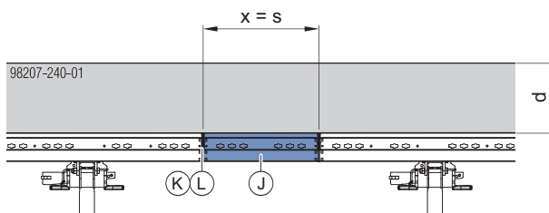
mit Tischelementen
