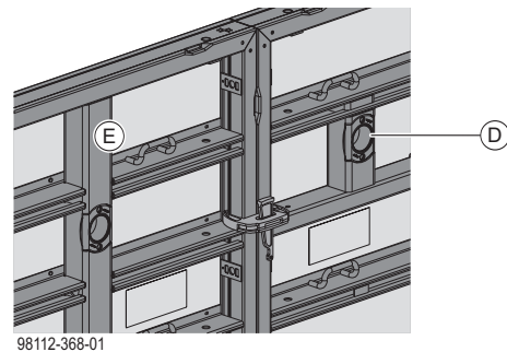
D Framax Xlife plus panel 0.90x3.30m (art. n° 589292600)
