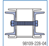
Schnitt A-A
