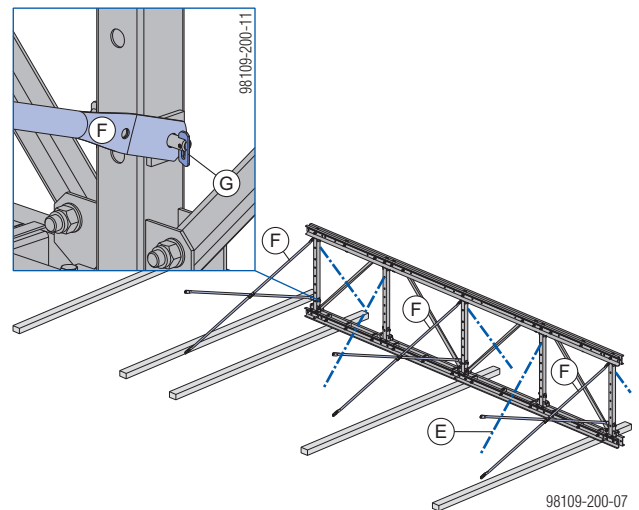
E Abstützung (bauseits)
