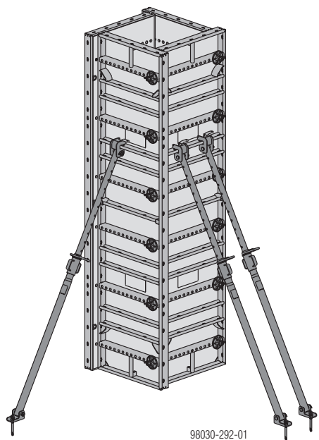
Prikaz s Frami Xlife-okvirnim elementom 3,00m.
