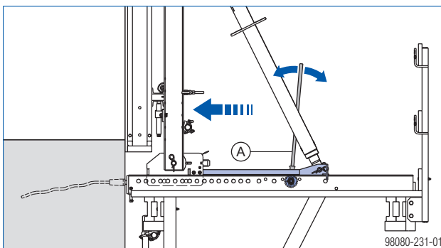
A Antriebsknarre MF 3/4" SW50
