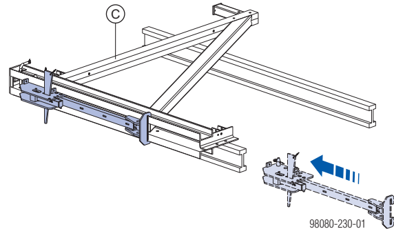
C Sperrenkonsole D22 F
