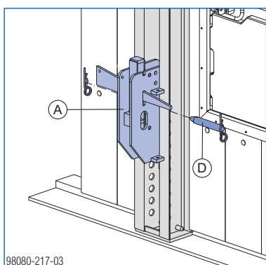
A Gelenkaufsatz D22
