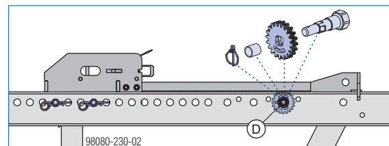
D Antriebs-Zahnrad
