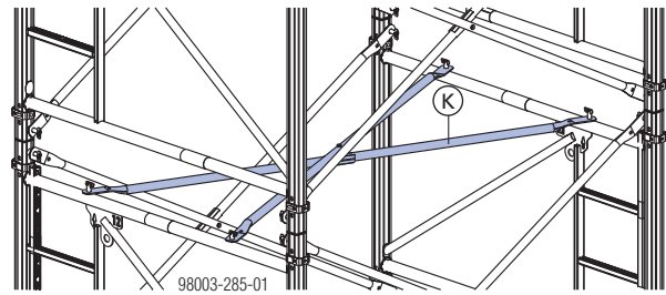
K Diagonalkreuz
