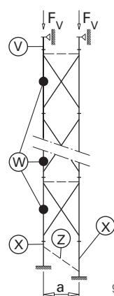
Плоскость раскосов
