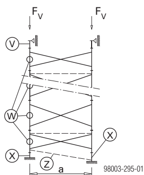
Плоскость раскосов
