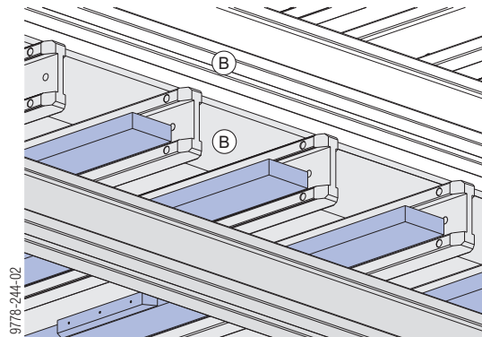
B Dokaflex-Tisch
