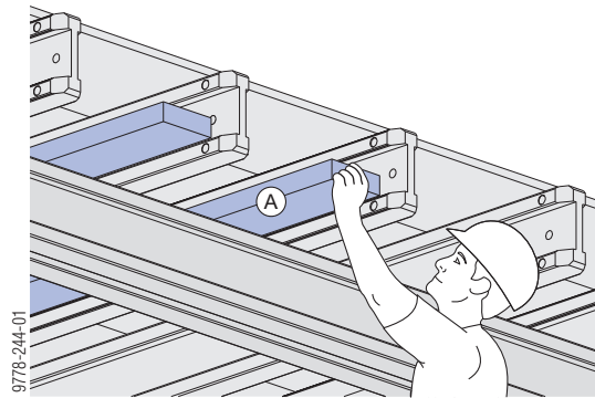
A Einschubträger
