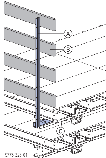
A Einschubgeländer T 1,80m
