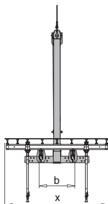
Tisch quer zur Gabel
