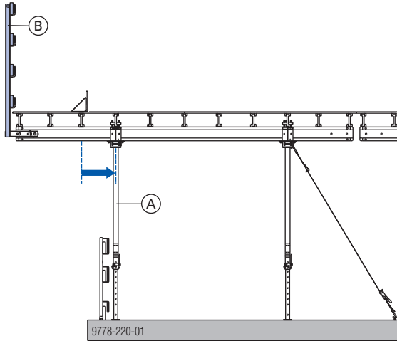
B Einschubgeländer T 1,80m bzw. Xsafe Seitenschutz XP
