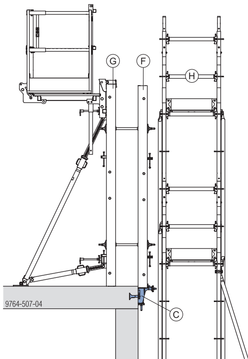
C Auflagewinkel Wandschalung 2G
