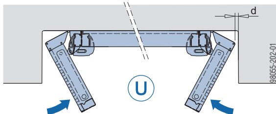
U Umsetzeinheit
