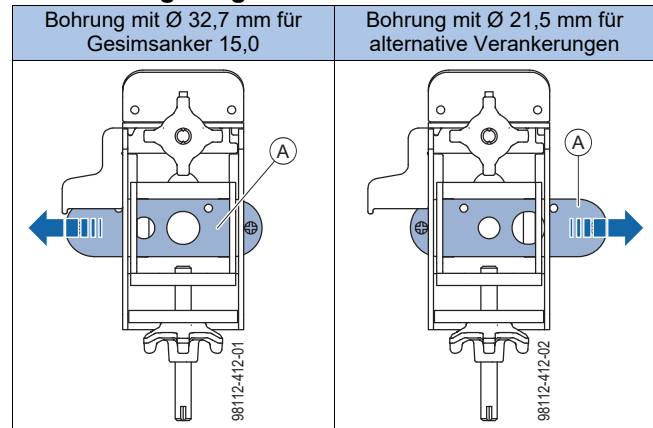
A Lasche zum Verschieben auf die jeweilige Bohrung
