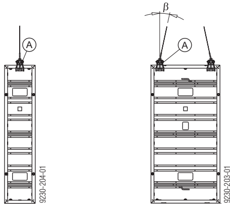
A Auflageblech
