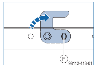
Einsatzstellung für Belag XBS
