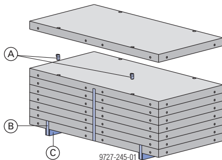
A Framax-Stapelkonus
