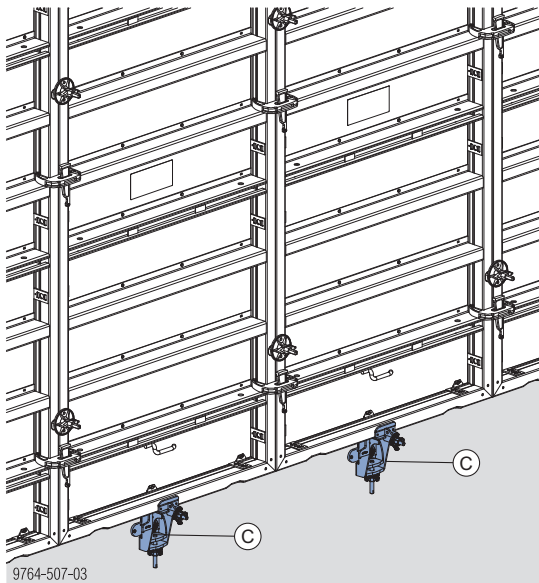
C Auflagewinkel Wandschalung 2G oder Auflagewinkel Wandschalung
