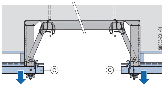
C Stirnabschalung
