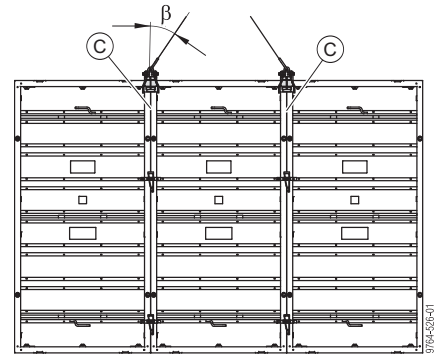
C Elementstoß
