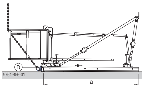
D Framax-Umsetzbügel
