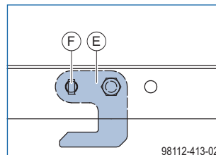
Parkstellung für Holzbohlen
