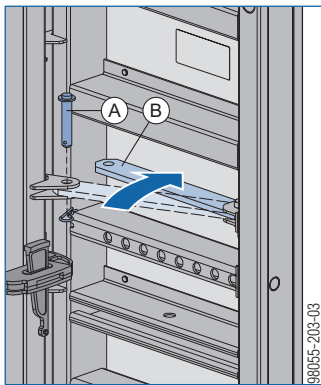
A Absteckbolzen B Lasche
