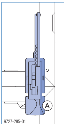
A Auflagerfläche am Profil
