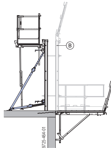
B Gegenschalung
