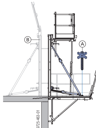
A Sternschraube
