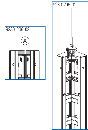
A Poziție de fixare: Profil interior al colțului interior
